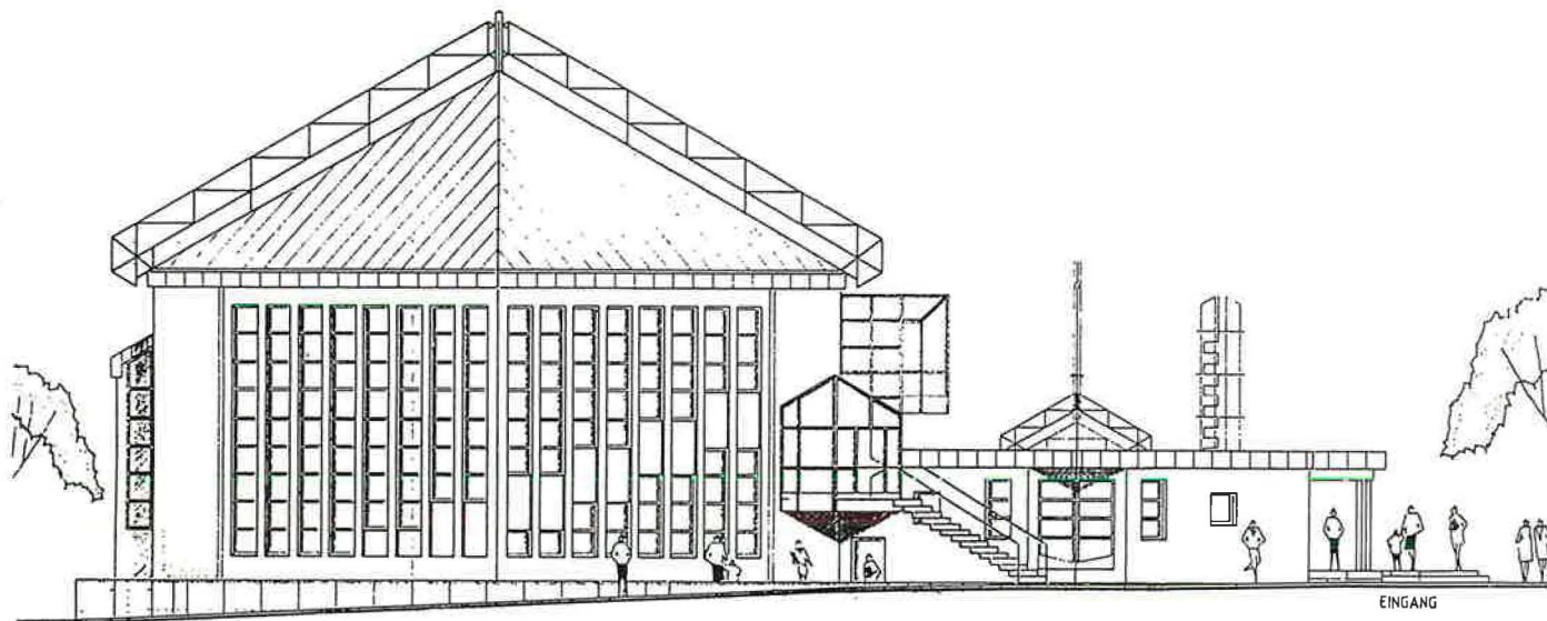
Südwest-Ansicht; M. 1 : 100
