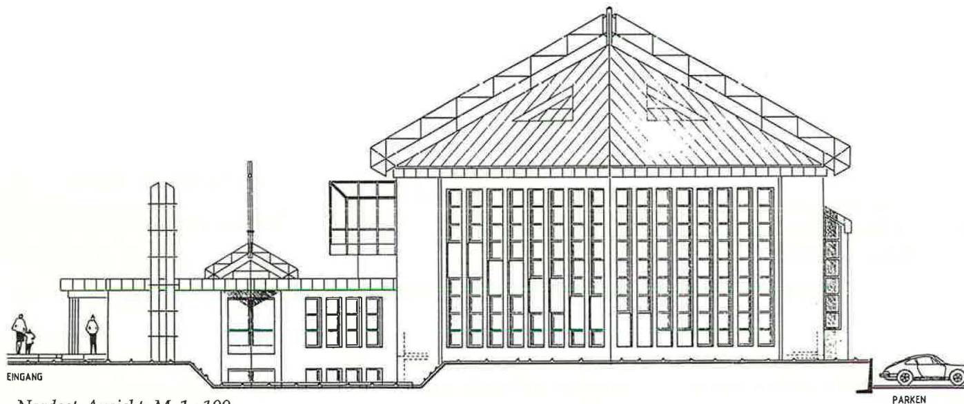
Nordost-Ansicht; M. 1 : 100
