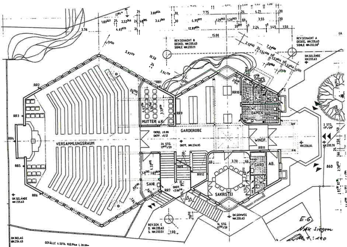
Grundriß
