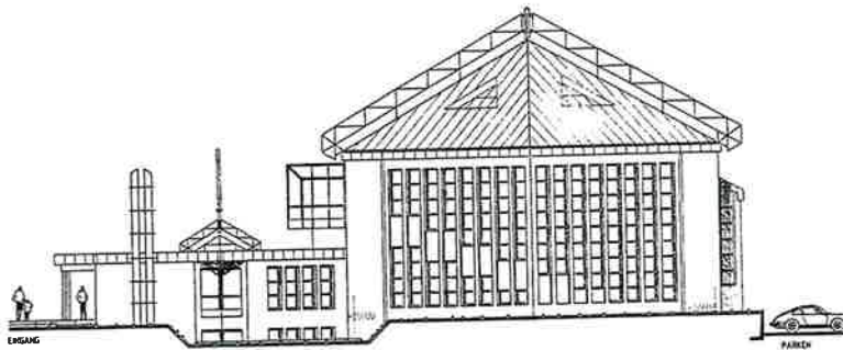
Nordost-Ansicht; M. 1 : 100
