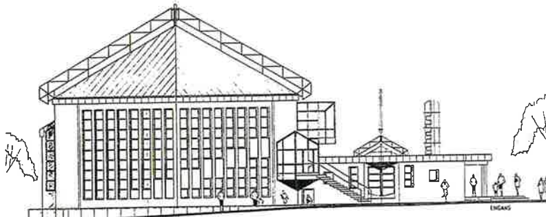
Südwest-Ansicht; M. 1 : 100
