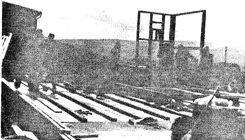
Montage der Fertigbauteile
