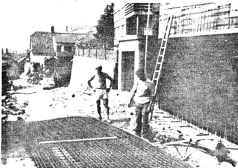
Bau der vorderen Stützmauer
