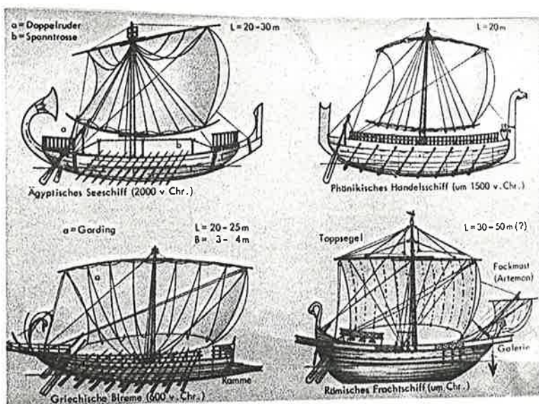
Schiffsmodelle aus verschiedenen Jahrhunderten. Unten rechts der Typ eines Schiffes, das der Apostel Paulus benutzt haben könnte
