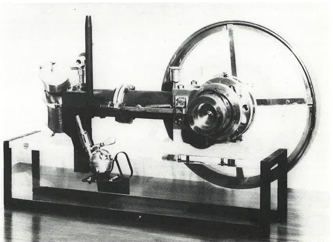
Erster 1/2 PS schnelllaufender Benzinmotor der Welt, von Maybach 1885 konstruiert
