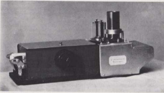
Die erste „Hostienbeträufelungsmaschine“, entwickelt von Bruder Bickelmann, Göppingen
